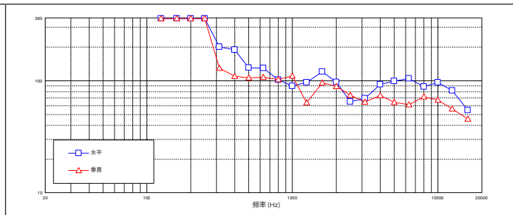
垂直离轴频率响应：
