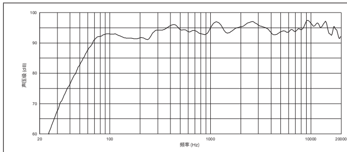
水平离轴频率响应：
