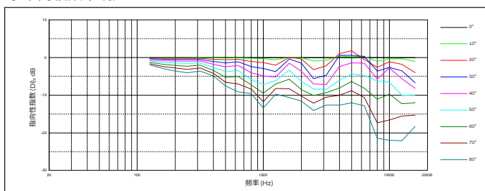
水平离轴频率响应：
